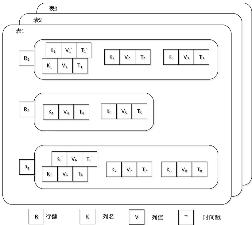
图 1 Key-Value 数据模型
